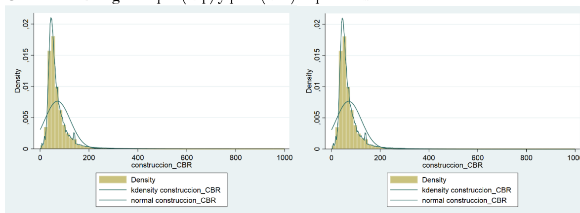
Gráfico I: Histograma pre (izq.) y post (der.) imputación
