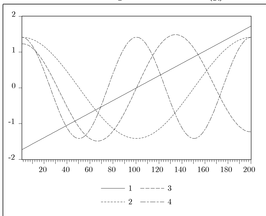
Polinomios Ortogonales de Chebishev ( g_i )
