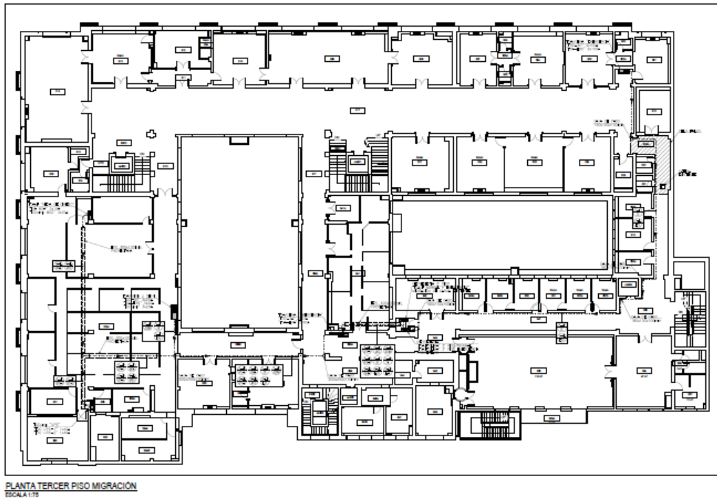
Figura 1: Plano de planta tercer piso con tendido de alimentadores proyectado
