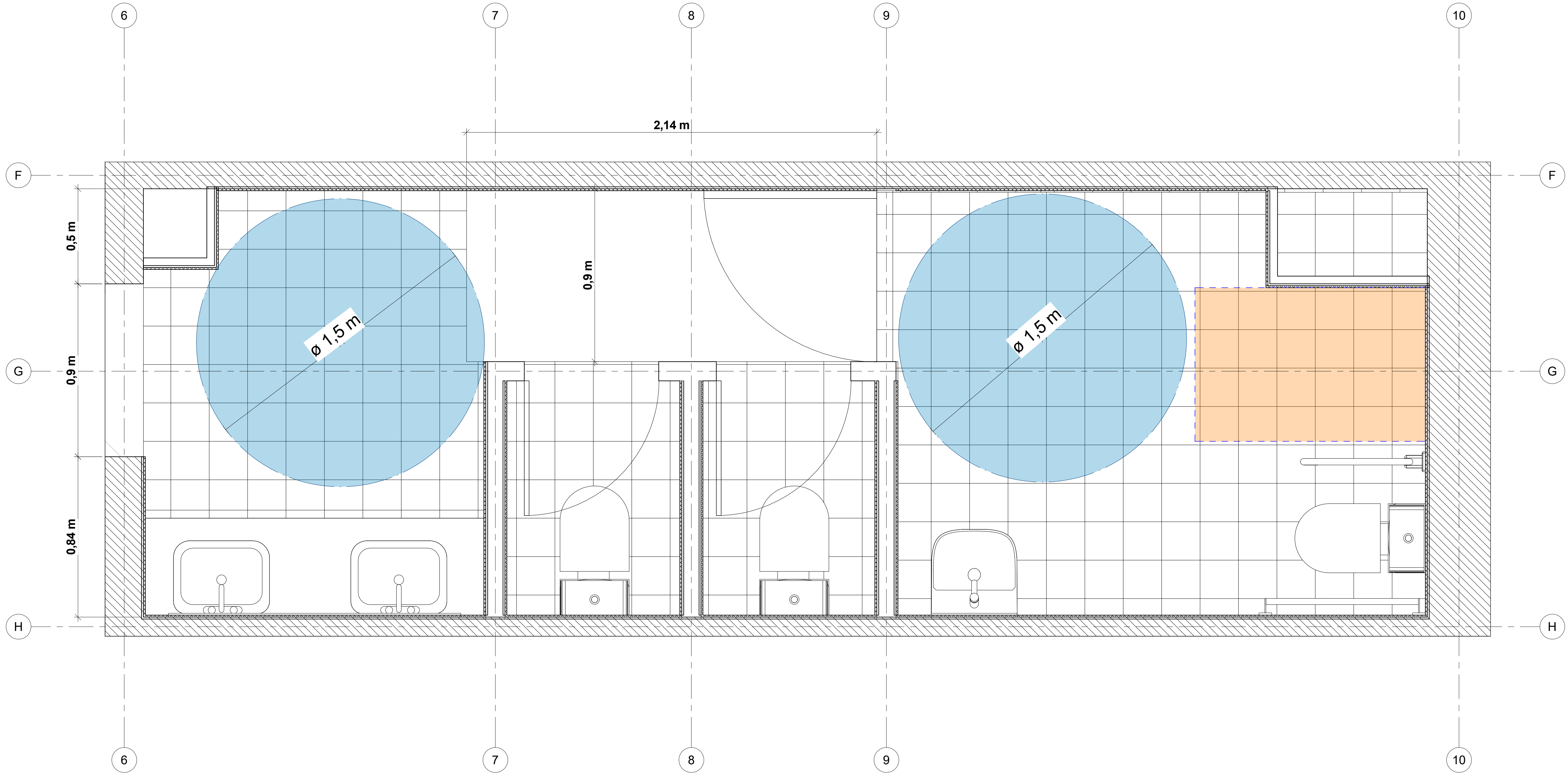
1 Planta Accesibilidad Universal 1:10
