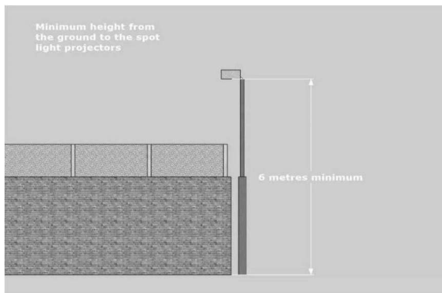
Figura 9 - Altura de luz
