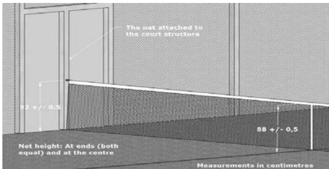
Figura 5 Altura neta
