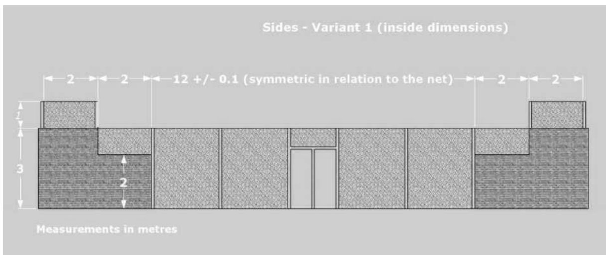
Figura 5 Tamaño lateral de la pista de pádel
